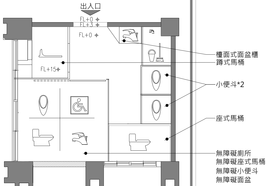
廁間平面配置圖 Toilet Plan
